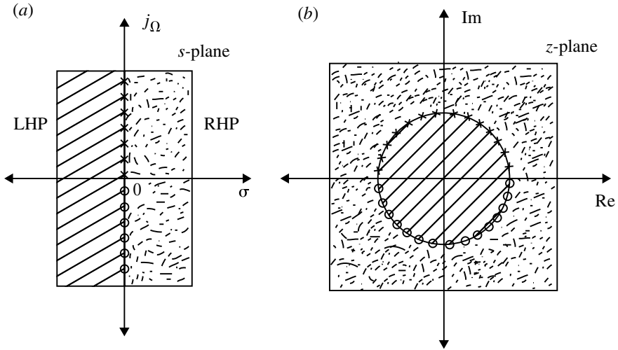
Fig. 4.3 s -plane to z -plane mapping
