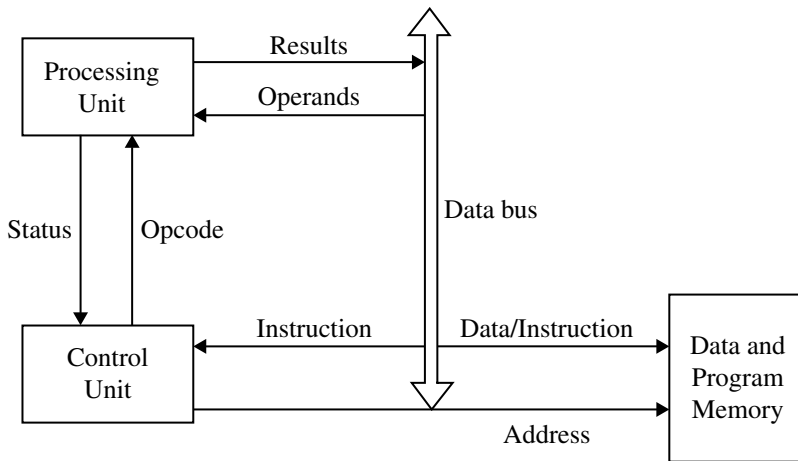
Fig. 6.2 Von Neumann architecture
