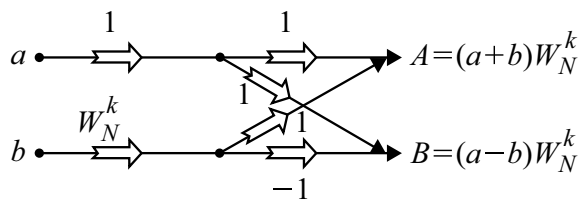
Fig. 3.66 Butterfly diagram for DIT radix-2 FFT
