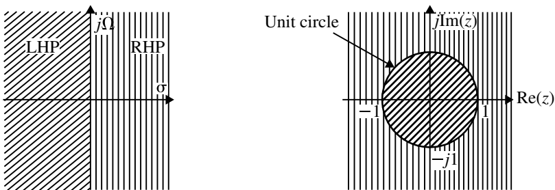
Fig. 4.63 Mapping of s -plane to z -plane
