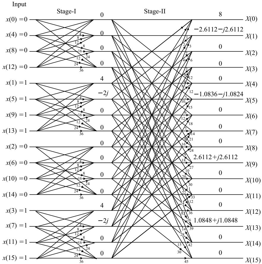
Fig. 3.45 Radix-4 DIT FFT algorithm for Example 3.46
